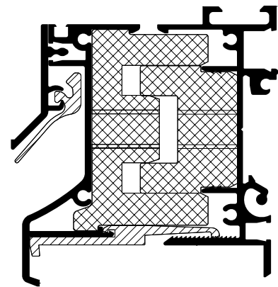
Vario-Air, schaal 1:2 Vario-Air, échelle 1:2
